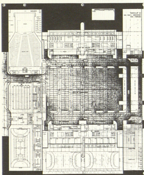
Planta +667,10
