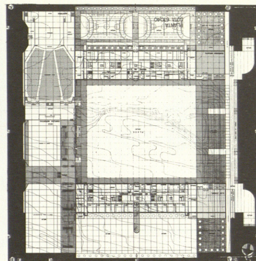
Planta +673,70
