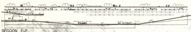
SECCION 2-2
